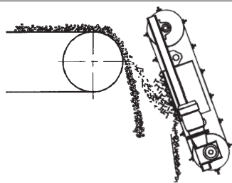
Posição 1 - LONGITUDINAL
